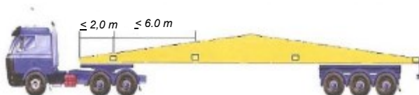
Figur 5 Sidomarkeringslykter och sidomarkeringsreflexer på sidan på mellanliggande last och längst bak på sidan på utskjutande last (2 kap. 9 §)
