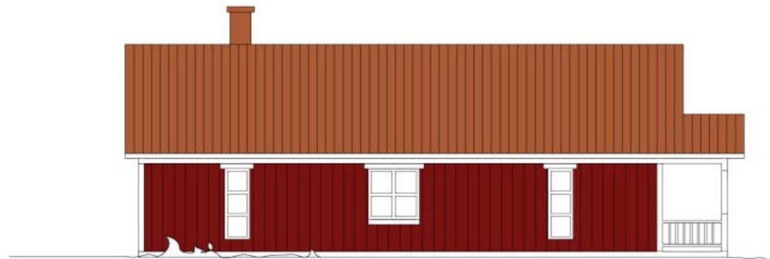
Fasad söder. Hus 9 Fasad norr. Hus 10
